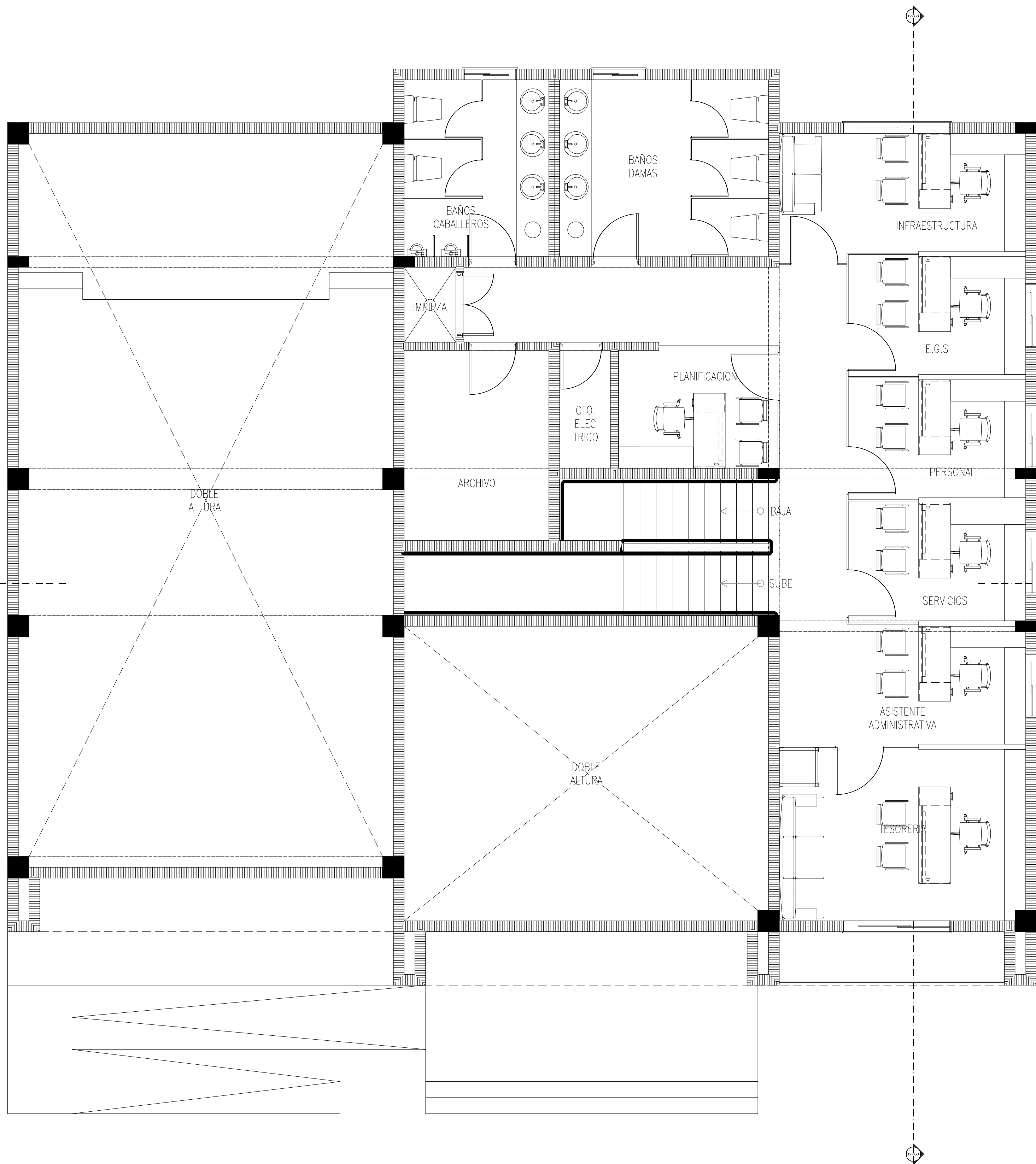
Planta Arquitectónica.- Esc. 1:50.- Nivel 2.-
