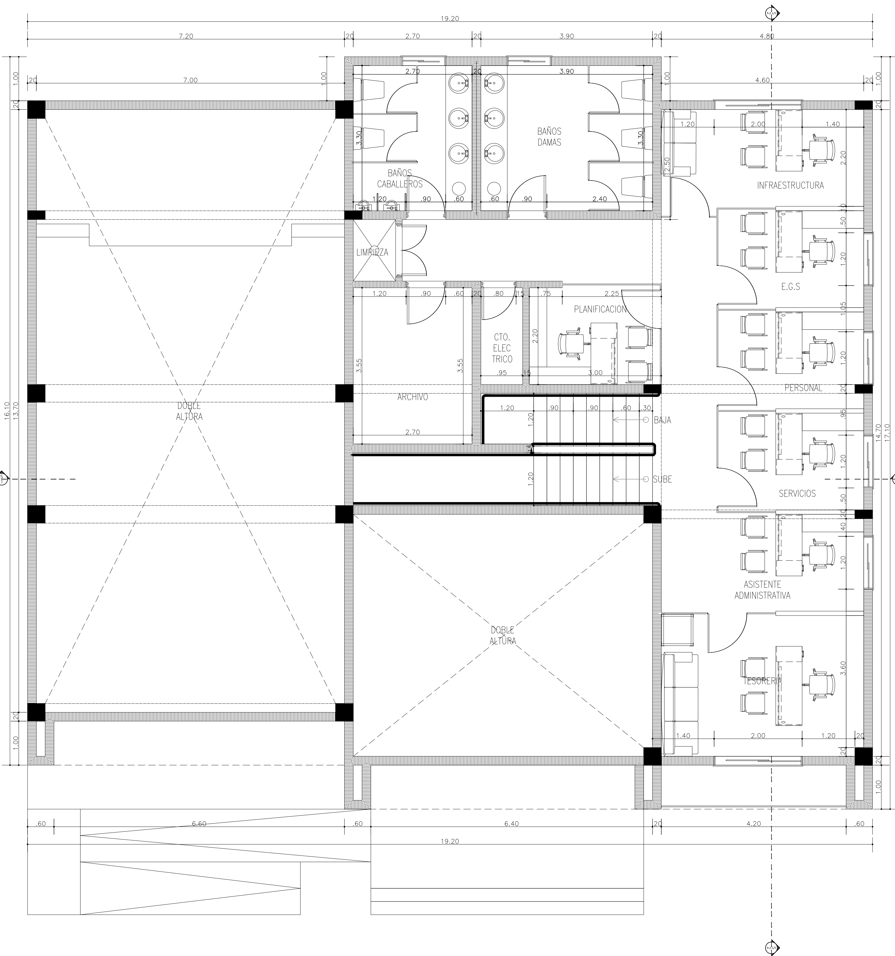
Planta Dimensionada.- Esc. 1:50.- Nivel 1.-
