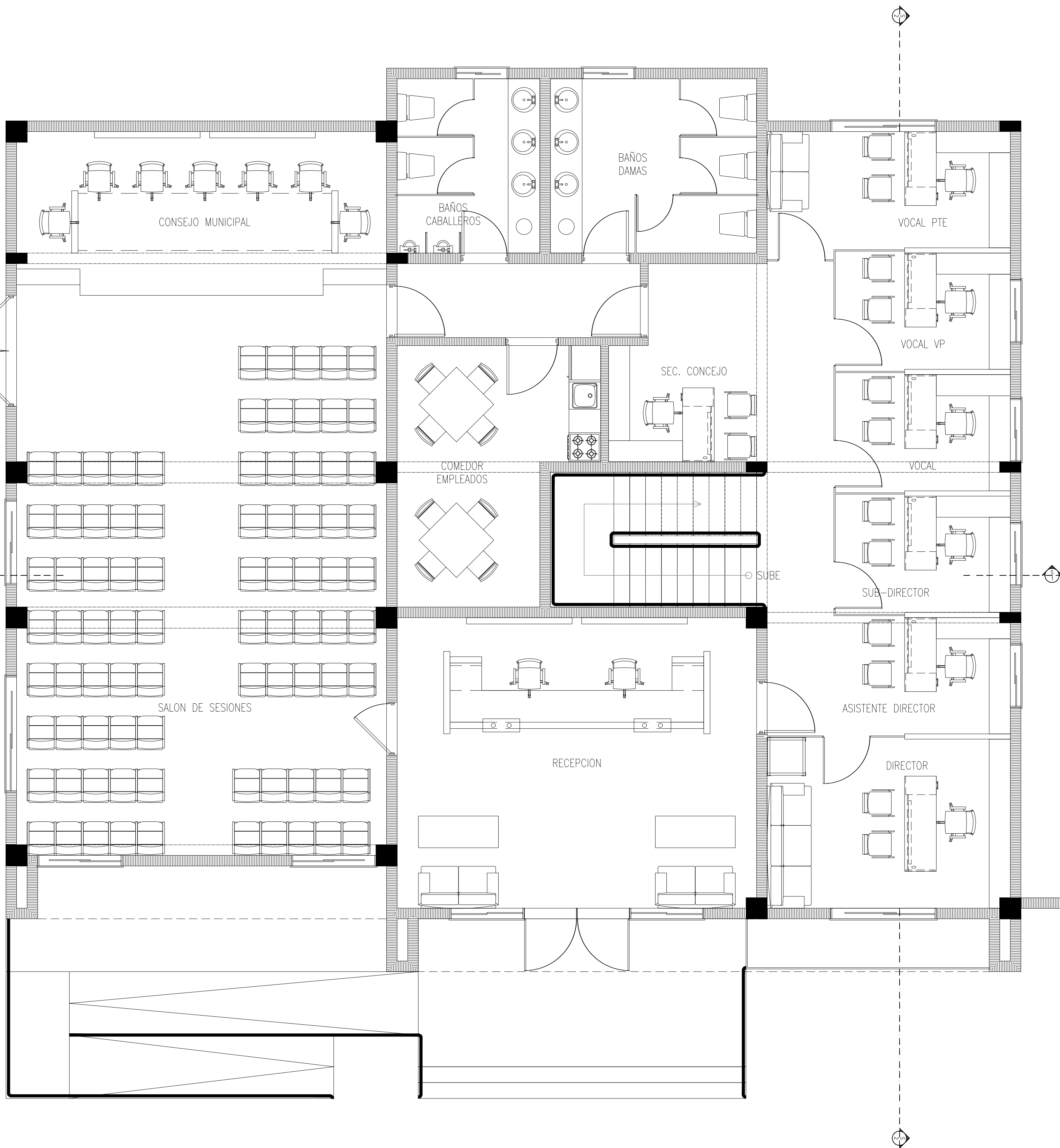
Planta Arquitectónica.- Esc. 1:50.- Nivel 1.-
